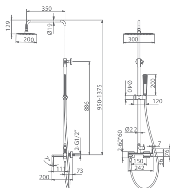
Barra "slim" de bañera de acero inox. S.304 redonda extensible. Rociador de acero inox. S.304 20x30 cm, extraplano y antical. Soporte mango de ducha regulable en altura. Mango de ducha redondo de 1 posición. Grifería monomando de latón con caño de bañera plegable. Distribuidor redondo. Caudal medio 12 l/min. Flexo 180cm. Cartucho monomando cerámico Ø28 mm.
