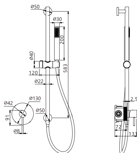
Barra de acero inox. S.304 redonda con toma de agua. Soporte mango de ducha deslizabile. Mango de ducha de 1 posición. Grifería monomando de latón. Caudal medio 10 l/min. Flexo 150cm. Cartucho monomando cerámico Ø35 mm.
