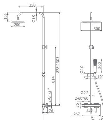
Barra "slim" de ducha de acero inox. S.304 redonda extensible. Rociador de acero inox. S.304 20x30 cm, extraplano y antical. Soporte mango de ducha regulable en altura. Mango de ducha redondo de 1 posición. Grifería monomando de latón con distribuidor incorporado. Caudal medio 12 l/min. Flexo 150cm. Cartucho termostático autolimpiable TURN CLEAN SYSTEM.
