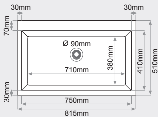
FREGADERO SOBRE ENCIMERA 1 seno rectangular MEDIDAS: 815 x 510 mm.
