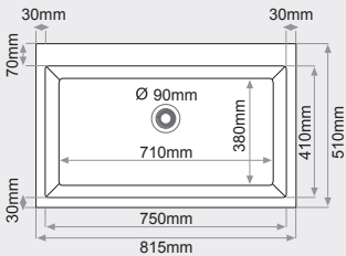
FREGADERO BAJO ENCIMERA 1 seno rectangular MEDIDAS: 815 x 510 mm
