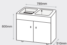
MUEBLE THOR MELAMINA MEDIDAS: 800x510x785mm.
