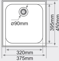
FREGADERO BAJO ENCIMERA 1 seno rectangular MEDIDAS: 375x450mm.
