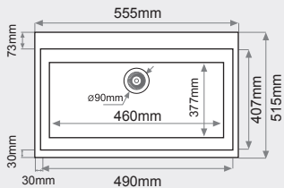
FREGADERO BAJO ENCIMERA 1 seno rectangular MEDIDAS: 555x515mm.
