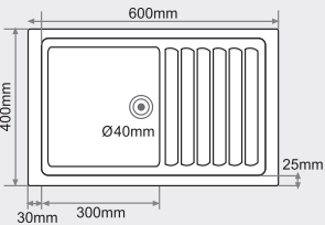
LAVADERO SOBRE ENCIMERA 1 lavadero + 1 escurridor MEDIDAS: 600x400mm.
