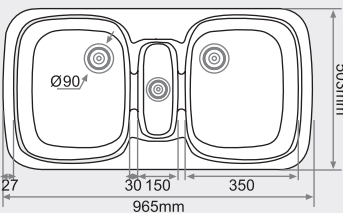
FREGADERO SOBRE ENCIMERA 2 senos + 1/2 cubeta MEDIDAS: 965x503mm.
