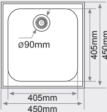
FREGADERO BAJO ENCIMERA 1 seno cuadrado MEDIDAS: 450x450mm.
