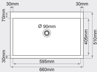
FREGADERO BAJO ENCIMERA 1 seno rectangular MEDIDAS: 660 x 510 mm
