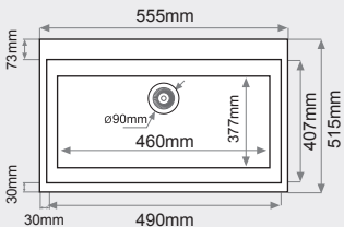
FREGADERO SOBRE ENCIMERA 1 seno rectangular MEDIDAS: 555 x 515 mm.
