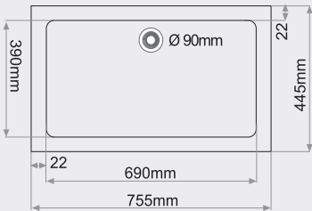
FREGADERO BAJO ENCIMERA 1 seno rectangular MEDIDAS: 755x445mm..
