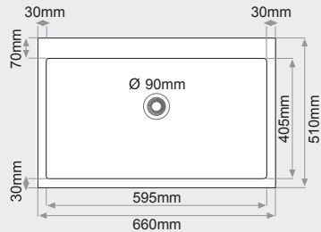
FREGADERO BAJO ENCIMERA 1 seno rectangular MEDIDAS: 660x510mm.
