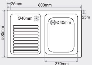
LAVADERO SOBRE ENCIMERA 1 lavadero + 1 escurridor MEDIDAS: 800x500mm.
