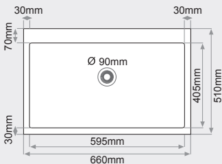
FREGADERO SOBRE ENCIMERA 1 seno rectangular MEDIDAS: 660 x 510 mm.
