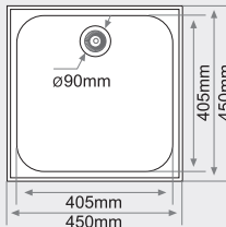
FREGADERO SOBRE ENCIMERA 1 seno cuadrado MEDIDAS: 450x450mm.
