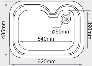
FREGADERO SOBRE ENCIMERA 1 seno rectangular MEDIDAS: 620x485mm.
