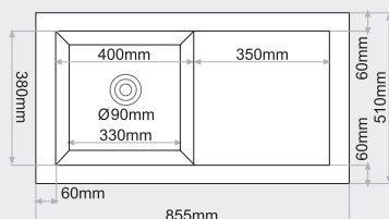
FREGADERO BAJO ENCIMERA 1 seno rectangular + 1 escurridor
