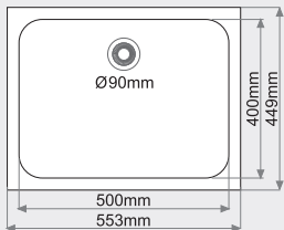
FREGADERO BAJO ENCIMERA 1 seno rectangular MEDIDAS: 553x449mm.
