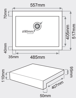
FREGADERO BAJO ENCIMERA 1 seno rectangular MEDIDAS: 557x517mm.
