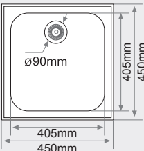
FREGADERO SOBRE ENCIMERA 1 seno cuadrado MEDIDAS: 450x450mm.
