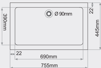
FREGADERO SOBRE ENCIMERA 1 seno rectangular MEDIDAS: 755x445mm.
