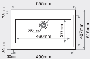
FREGADERO BAJO ENCIMERA 1 seno rectangular MEDIDAS: 555 x 515 mm
