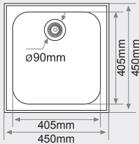
FREGADERO BAJO ENCIMERA 1 seno cuadrado MEDIDAS: 450x450mm.
