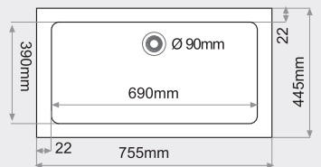
FREGADERO BAJO ENCIMERA 1 seno rectangular MEDIDAS: 755x445mm.
