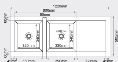
FREGADERO BAJO ENCIMERA 2 senos rectangulares + 1 escurridor
