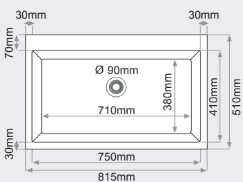
FREGADERO BAJO ENCIMERA 1 seno rectangular MEDIDAS: 815x510mm.
