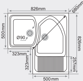
FREGADERO SOBRE ENCIMERA 2 senos angulares MEDIDAS: 826x826mm.
