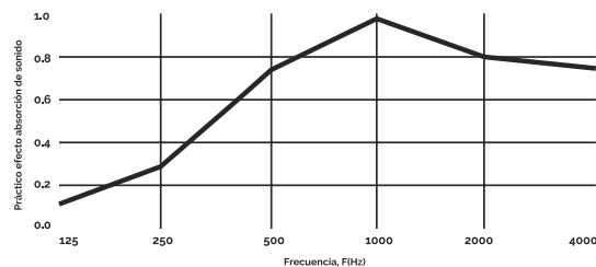
Instalación directa a pared
