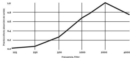
Instalación con listones de 45 mm y lana mineral
